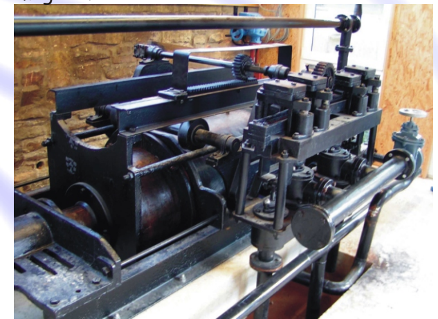
Lambach-Pumpe (Wassersäulenmaschine)
