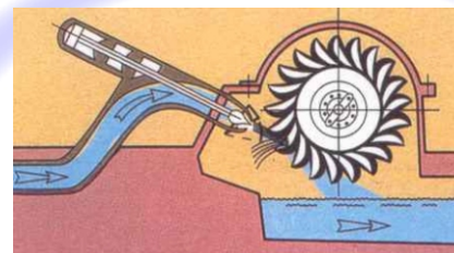
Schema einer Pelton-Turbine
